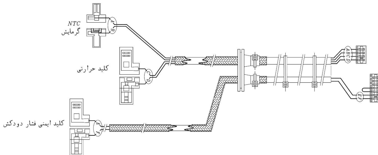
130-17: مجموعه سیم محفظه احتراق Parma 22Rsi IR
