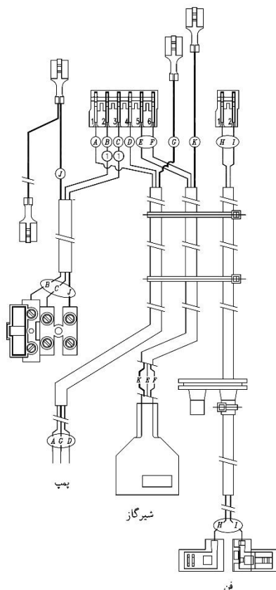
130-14: مجموعه سیم ولتاژ بالا Bita 22Sealed IR
