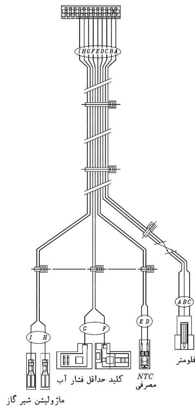
130-15: مجموعه سیم ولتاژ پایین Bita22 Sealed IR
